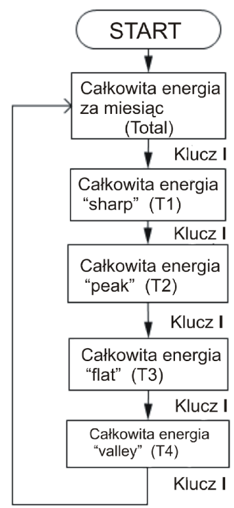
Rys 18. selekcja multi-taryfy
