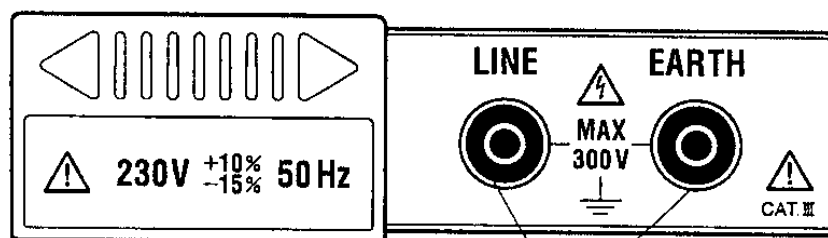
Gniazda wejściowe przewodów pomiarowych testu izolacji i ciągłości przewodu ochronnego
